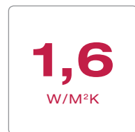
Toplotna prevodnost
